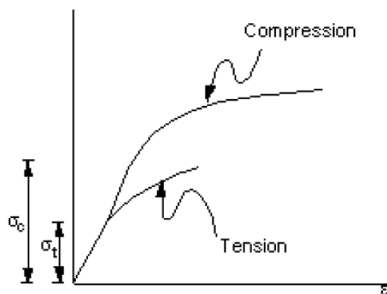
شکل ۷ پلاستیسیته چدن
