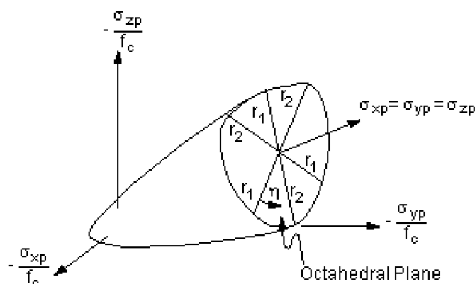
تصویر (پ-الف-۱): سطح گسیختگی سه بعدی در فضای تنش‌های اصلی
