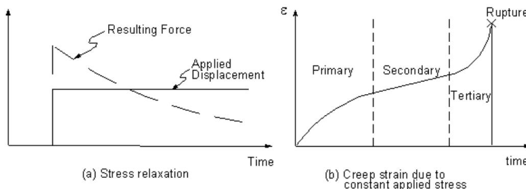
شکل ۸ آزاد سازی تنش و خزش
