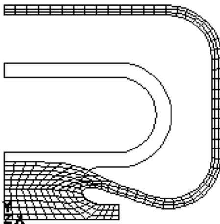
شکل ۱۳ سازه هایپر الاستیک
