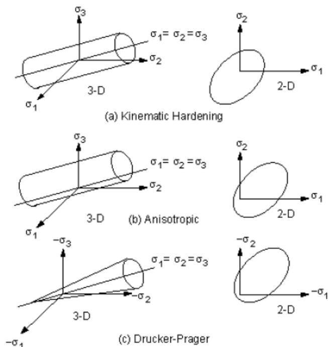
شکل ۲ سطوح جاری شدنگی برخی مصالح غیر خطی
